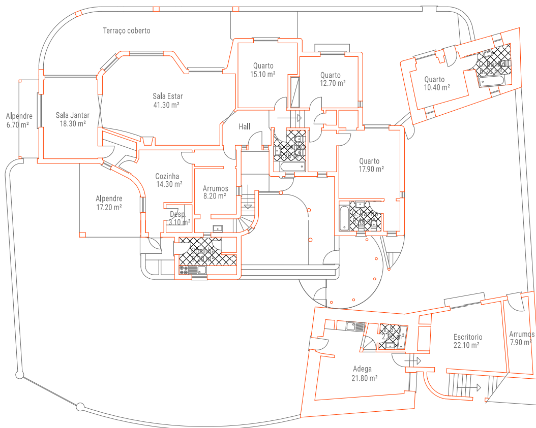
PLANTA DO R/CHÃO
